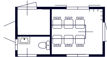
wagen 8 215x400
