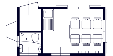
wagen 10 215x400
