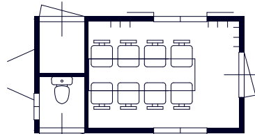
wagen 7 215x400
