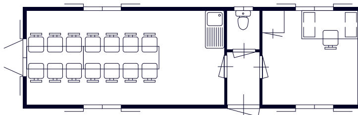
wagen 28 250x900
